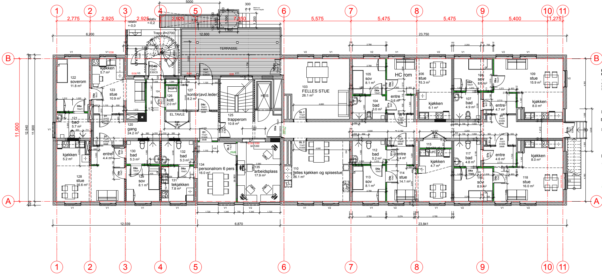
PLAN 1.etasje
