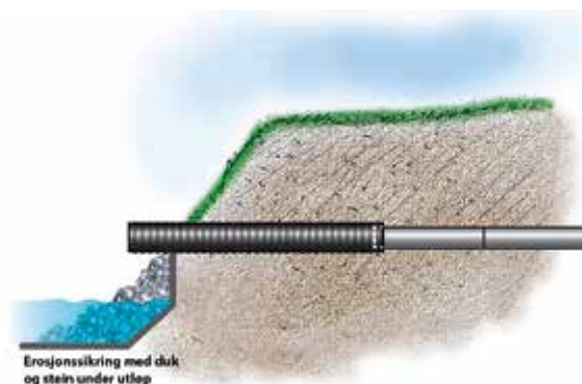
Figur 19: Nytt, minst 6 meter langt utløpsrør i plast kobles på gammel ledning.
