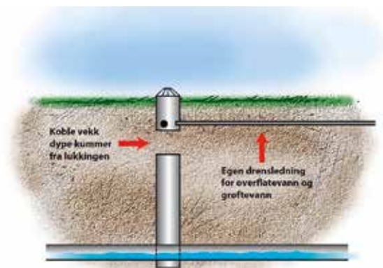
Figur 8c: Dersom en har svært dype kummer som det eroderer rundt, kan det være nødvendig å koble dem vekk for å sikre mot videre erosjon.
