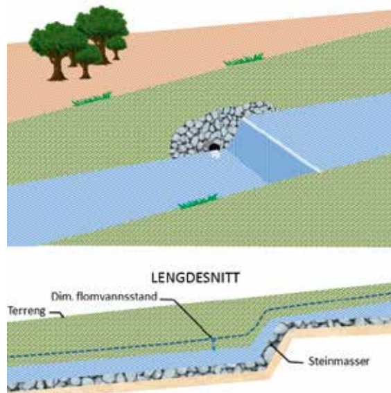
Figur 7: For å holde farten nede kan en anlegge stryk som virker som energidreper. Det er viktig at disse erosjonssikres godt med steinsetting.
