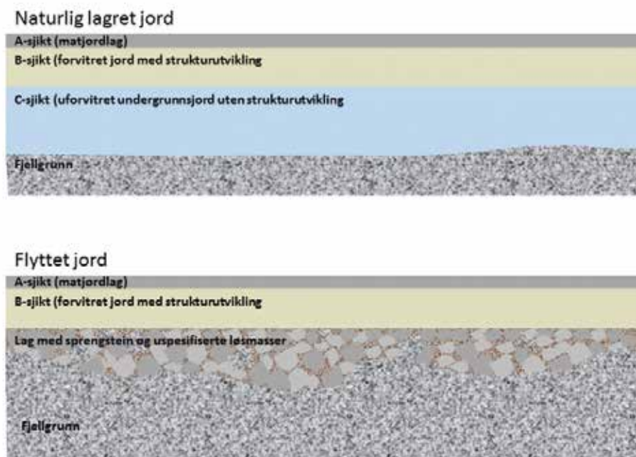
Figur 21: Prinsippkisse som viser oppbygging av jordprofilen før og etter jordflytting.
