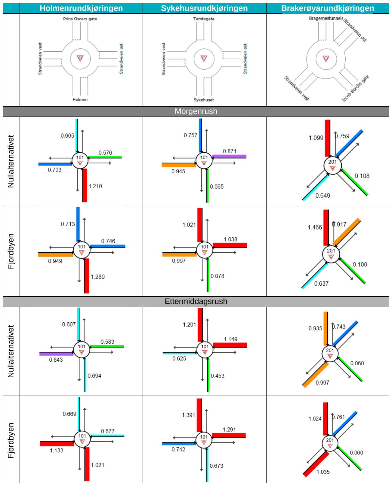
Figur V- 20: Kapasitet i kryss i Nullalternativet og med Fjordbyen
