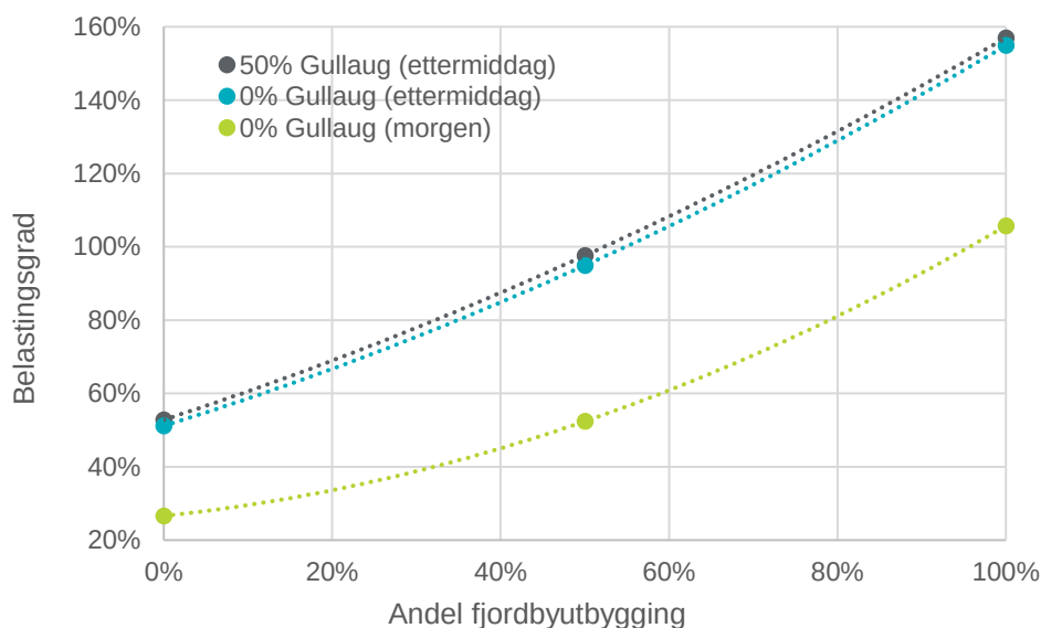
Figur 6-9 Belastningsgrad i rundkjøringen avhengig av ulike andeler utbygging i Fjordbyen og Gullaug
