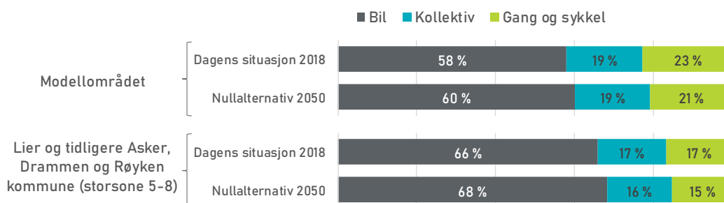
Figur 4-2: Reisemiddelfordeling for 2018 og 2050 for modellområdet og for området Lier og tidligere Asker, tidligere Drammen kommune og Røyken kommune (storsone 5-8).
