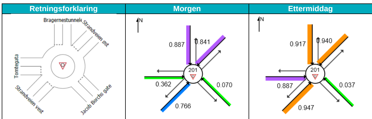
Figur 3-6: Belastningsgrad i Brakerøyarundkjøringen i dagens situasjon.
