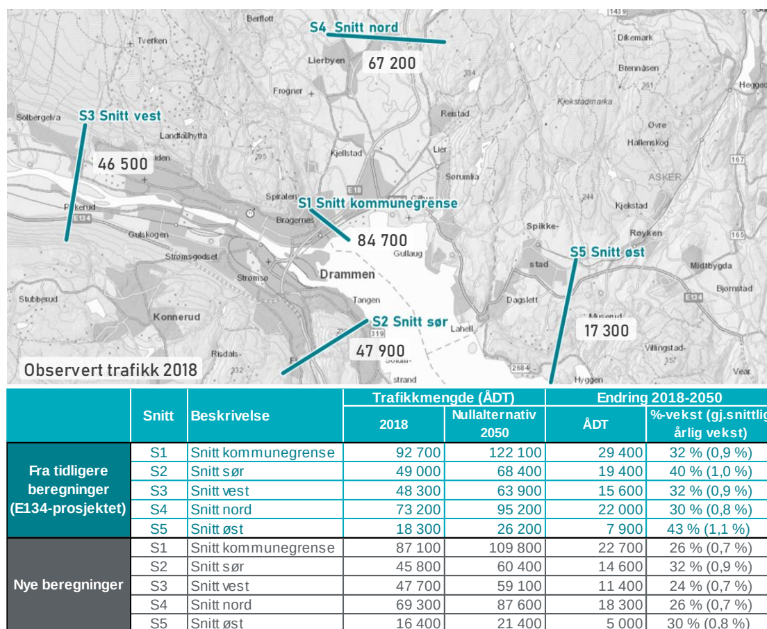
Figur V- 2: Observert trafikk over snitt i 2018 og beregnet trafikk over snitt i 2018 og 2050, samt endringen i trafikkmengde fra 2018 til 2050. Tidligere beregninger (E134-prosjektet) i turkis og nye beregninger i grå.
