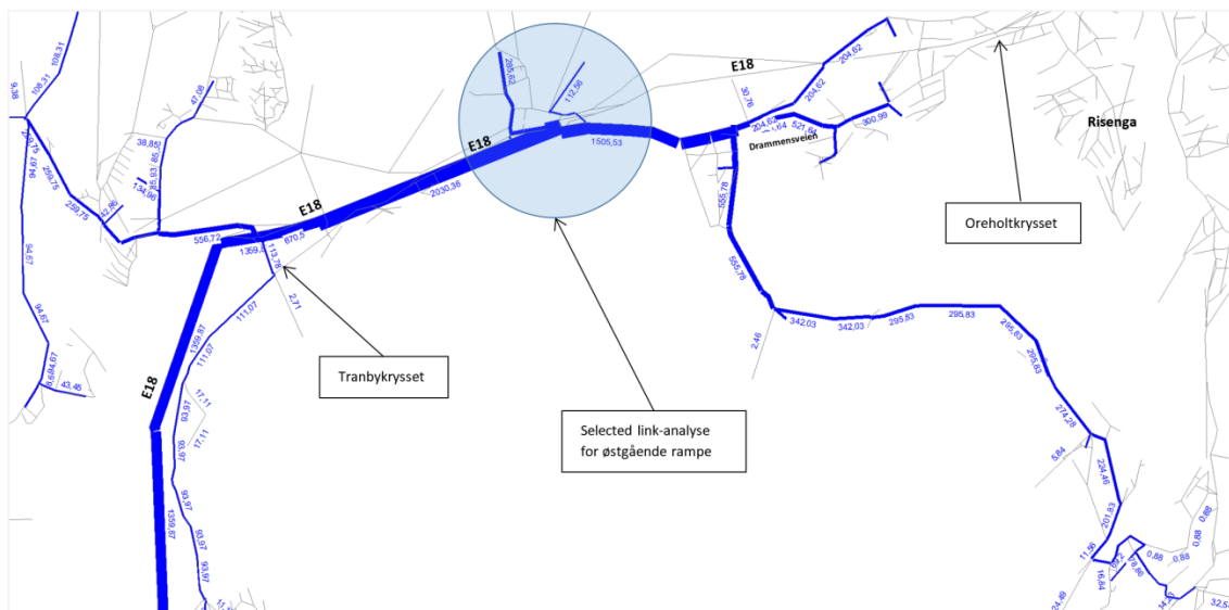
Figur 57. Selected link-analysis for trafikk på ny østgående rampe for kryss mellom E18 og fv. 16
