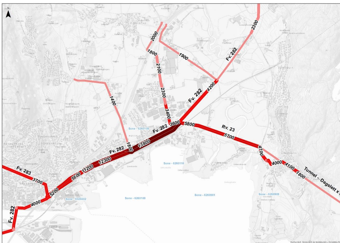
Figur 7. Differanseplott som viser endring i antall kjøretøy/døgn mellom scenario 2 (BBP2 + Lierstranda + Gullaug) og scenario 0B (BBP2). Rødefarge angir økning i trafikkvolum.
