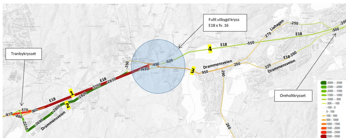
Figur 45. Differanseplott som viser endring i antall kjøretøy/døgn ved åpning av vestgående og østgående ramper i krysset E18 x fv. 16. Røde tall angir økning og grønne tall angir nedgang i trafikkvolum.
