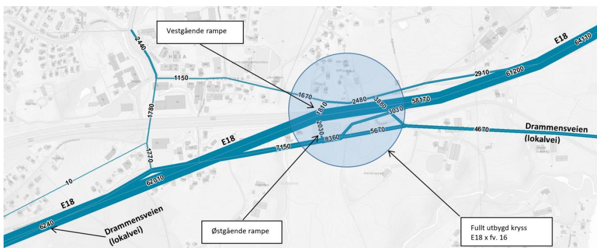
Figur 34. Beregningsresultater fra RTM (Antall kjøretøy/døgn - ÅDT 2030 med fullt utbygd kryss E18 x fv. 16 Drammensveien)
