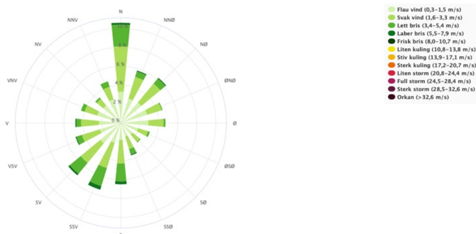
Vindrose for E18 Lierskogen (SN19923) i perioden; 9.2015–10.2024.
