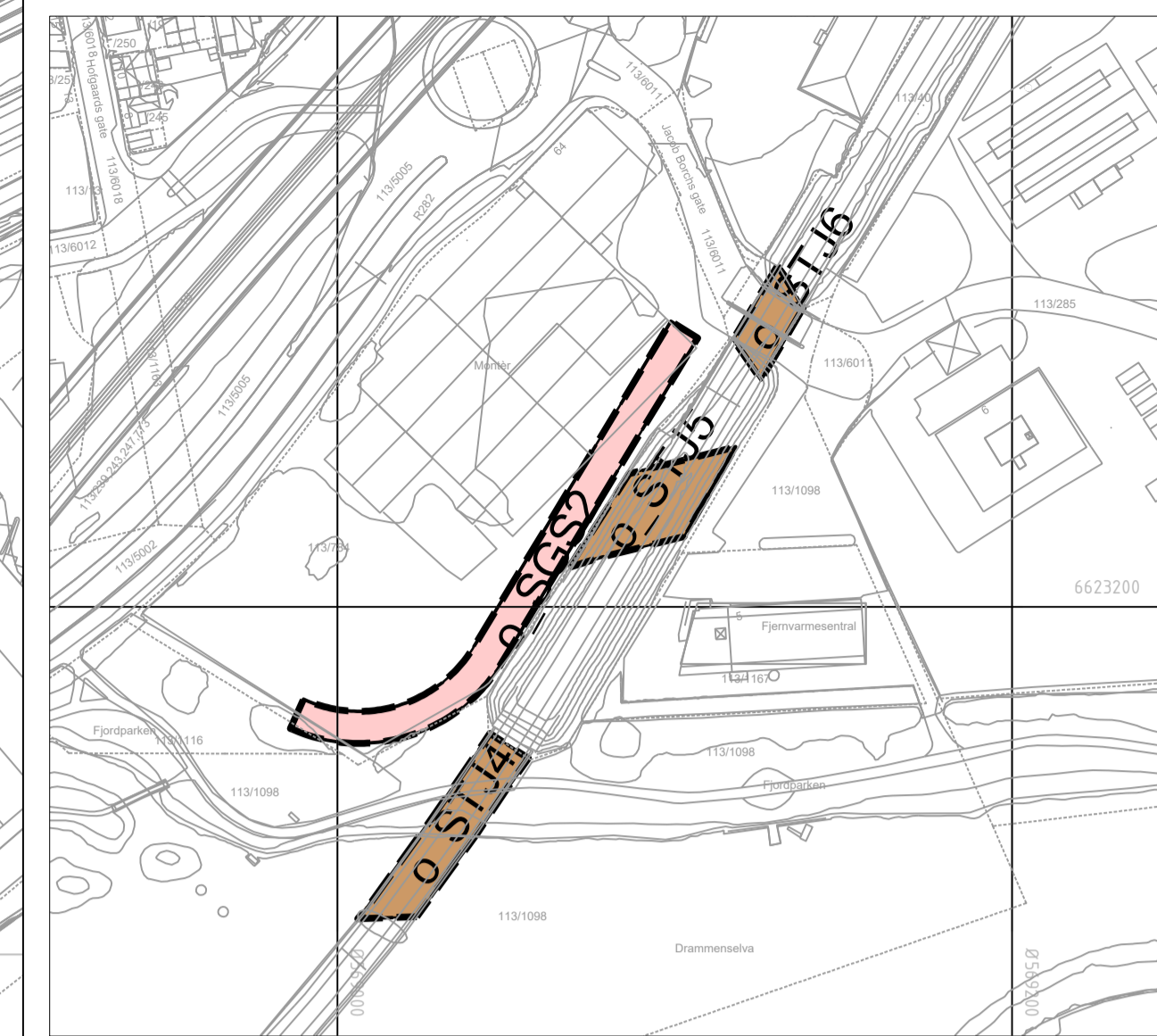
Vertikalnivå 3 Kartmålestokk: 1:2000
