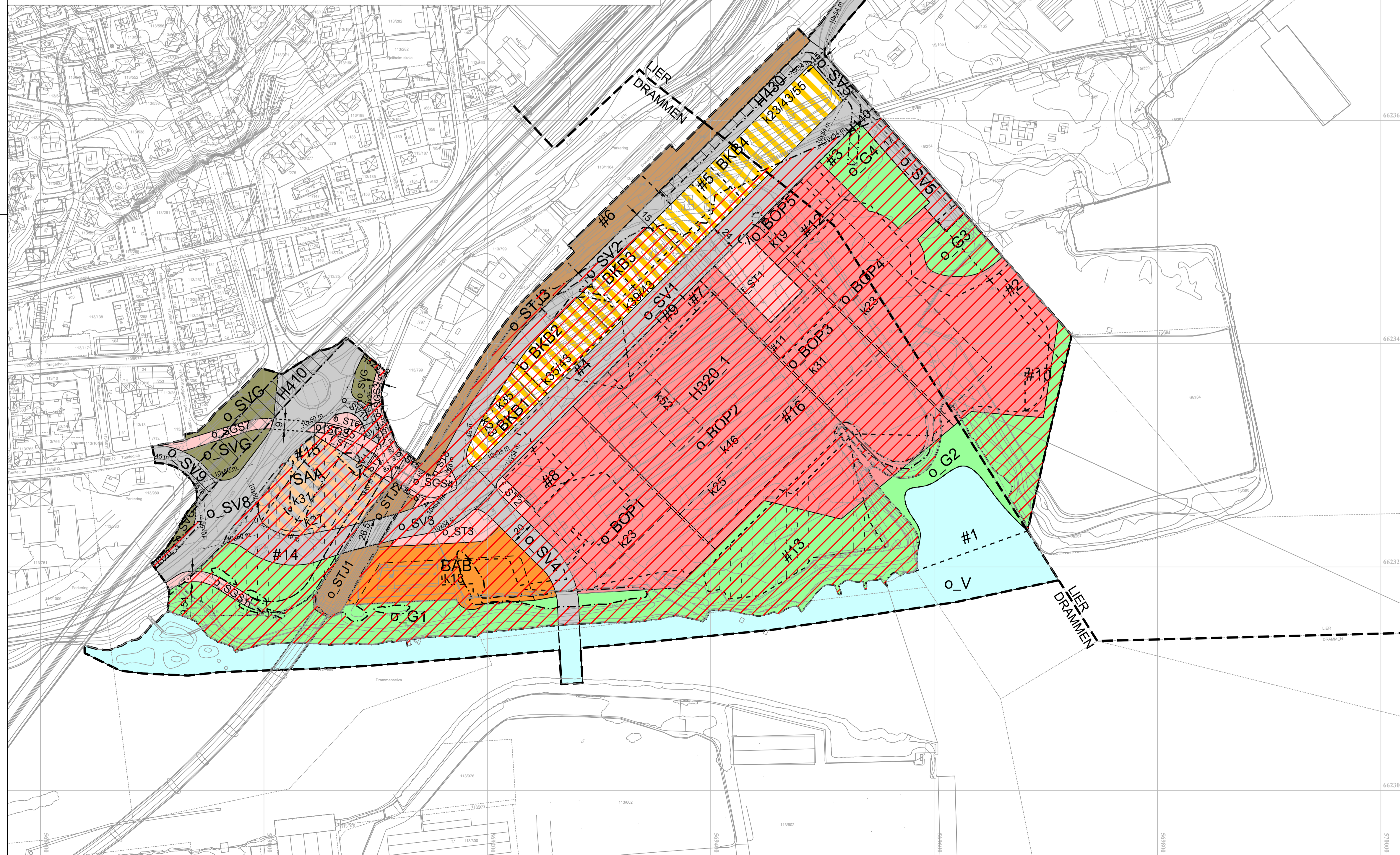
Vertikalnivå 1, Kartmålestokk: 1:2000
