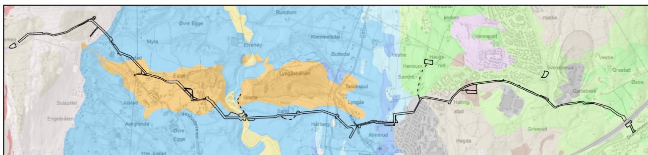
Figur 9 Løsmassekart fra NGU. Rosa er tynt løsmassedekke over berg, blått marine avsetninger, oransje breelvavsetninger, gul elveavsetninger og grønt morene.
