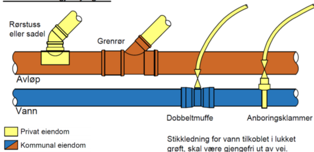
Grensesnitt i gjenfylt grøft
