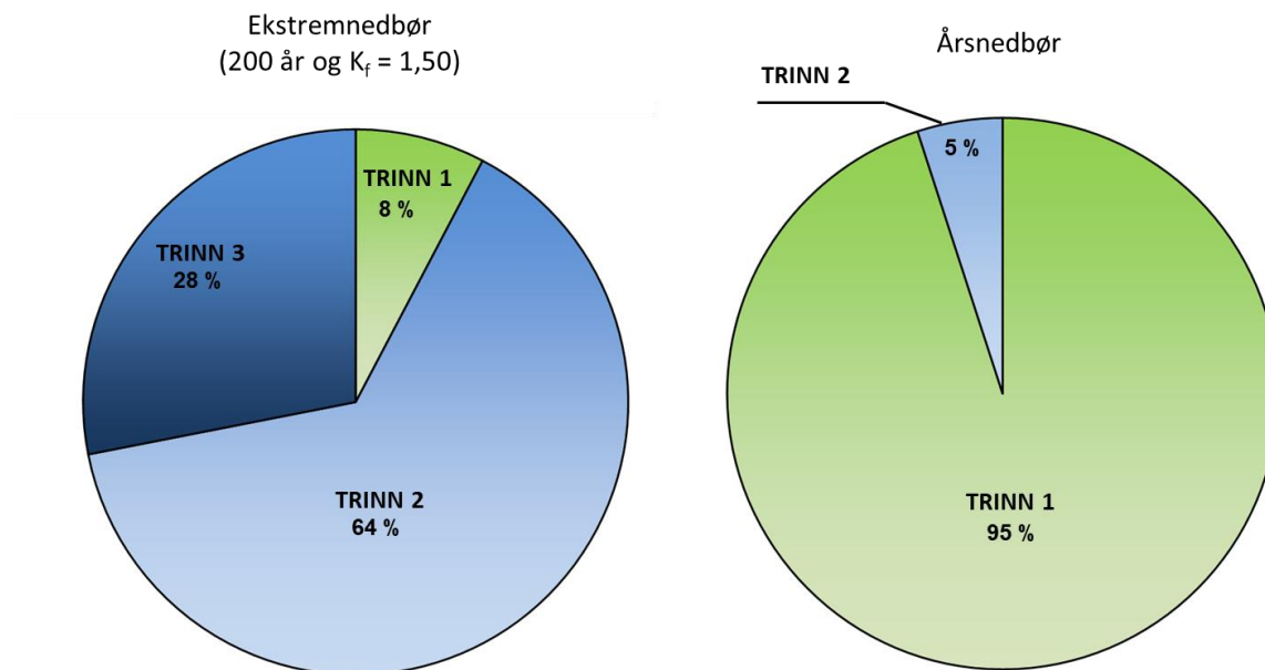
Figur 4: Fordeling av nedbørmengder per trinn for ekstremhendelse (200 år med klimafaktor 1,50) og over året. Dimensjoneringskriterie for Trinn 2 er 20 års gjentakintervall med klimafaktor på 1,50. Nedbørstatistikk fra Asker målestasjon er benyttet og verdier er beregnet ved å ta gjennomsnitt av fordelinger for regnvarigheter mellom 10 og 1440 minutter.
