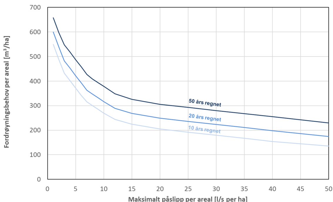
Figur 3: Nødvendig fordrøyning per areal som funksjon av gjentakintervall og maksimalt påslipp til offentlig nett. Forutsetninger for beregningene er IVF-statistikk fra Asker, klimafaktor på 1,40, midlere avrenningskoeffisient på 0,60 og at midlere utløp fra fordrøyningsløsningen under regnhendelsen er 70 % av maksimalt påslipp. Med fordrøyningsvolum menes det volum som både kan lagres og infiltreres under regnhendelsen.
